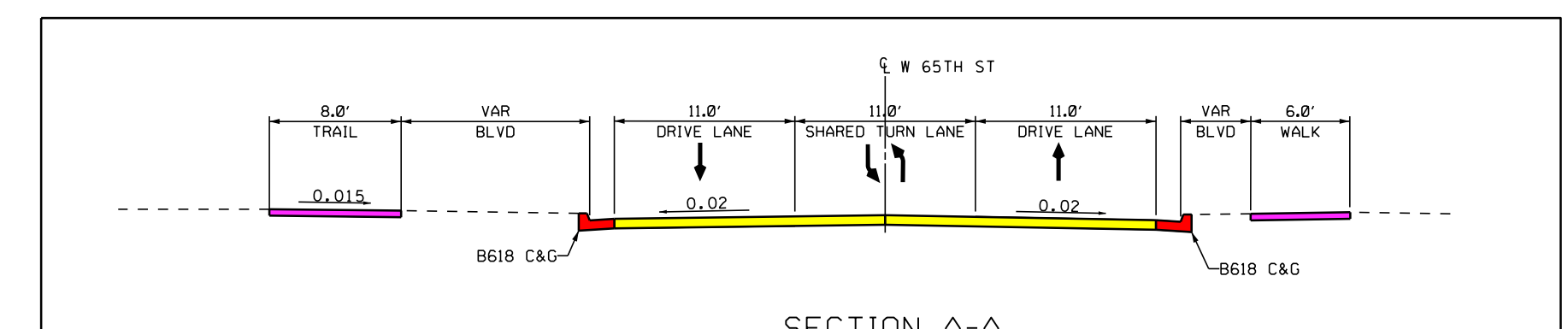
SECTION A-A
